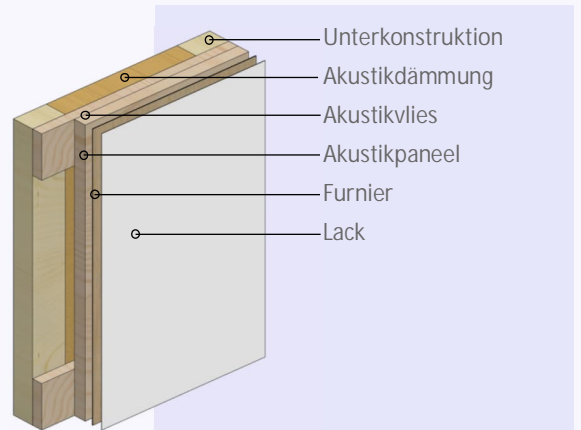
Die Unterkonstruktion besteht aus Holz- und Metallteilen. Die Akustikdämmung kann aus Mineralwolle, Polyester- oder Holzfasern bestehen. Zudem ist ein Akustikvlies vorhanden. Das Akustikpaneel kann aus Sperrholz, MDF oder Massivholz gefertigt sein und ist furniert oder mit Schichtstoff belegt. Abschließend ist es fertig lackiert.
